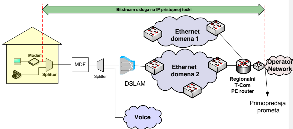
Slika 16. Veleprodajni širokopojasni pristup za pružanje VoIP usluge na IP razini u slučaju kada krajnji korisnik ostvaruje Osnovni pristup mreži putem usluge HT-a
